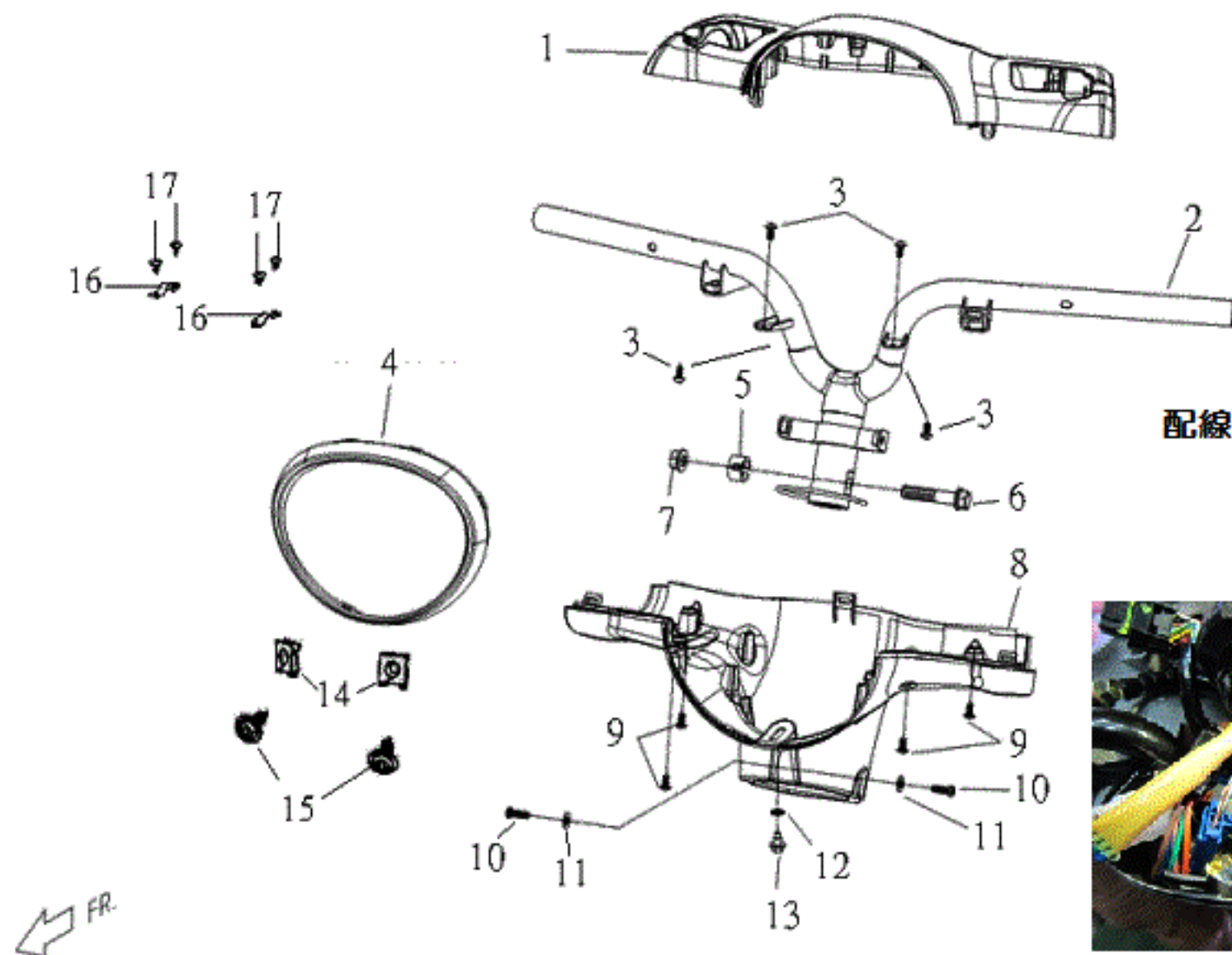
F1 方向把手前後蓋、方向把手管 COVER FR&RR, HANDLE BAR.
